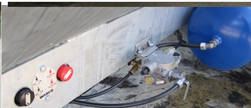
Trykluftbremser
